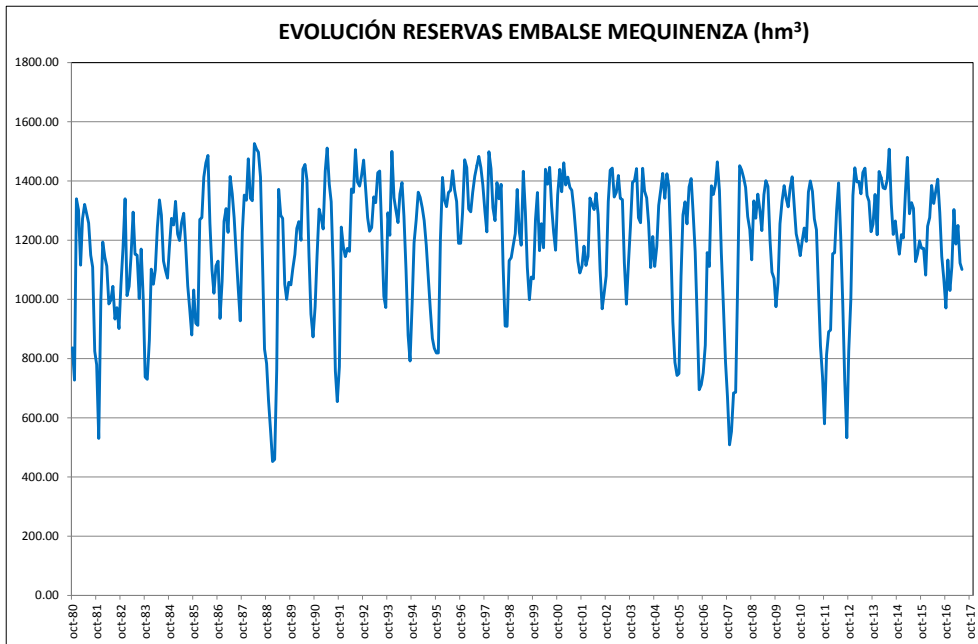
Figura 3. Evolución de las reservas del embalse de Mequinenza
