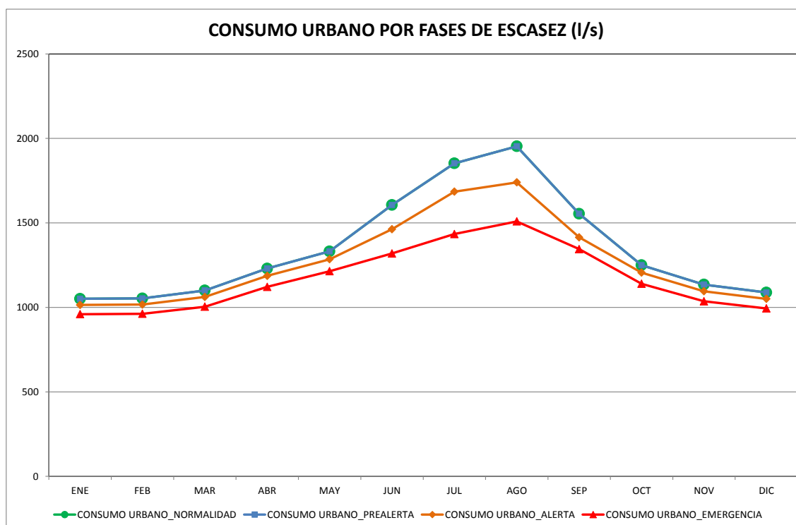
Figura 18. Consumo uso urbano por fases de escasez (l/s)
