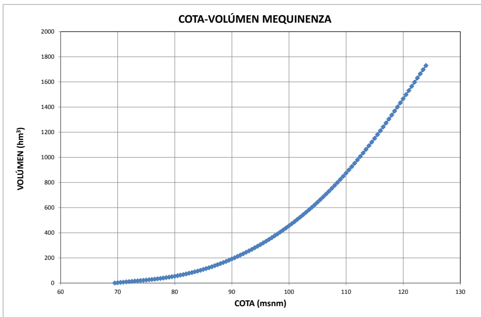
Figura 4. Gráfico Cota-Volumen embalse de Mequinenza
