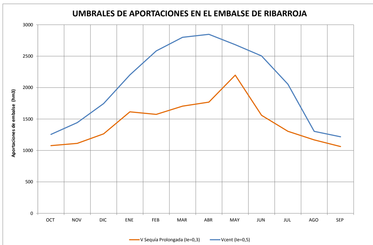
Figura 22. Umbrales de aportaciones en el embalse de Ribarroja
