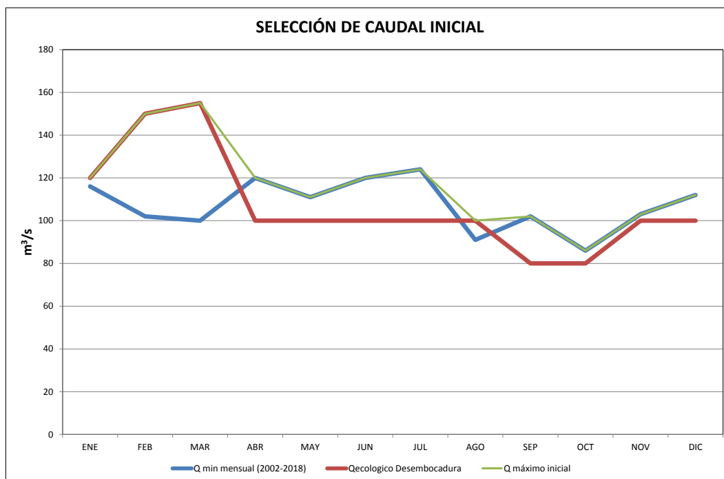
Figura 26. Selección caudal inicial Estación de Aforo EA-163
