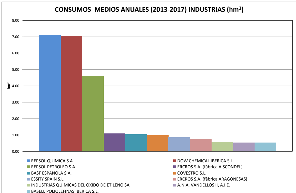
Figura 8. Consumos de industrias > 0,5 hm 3
