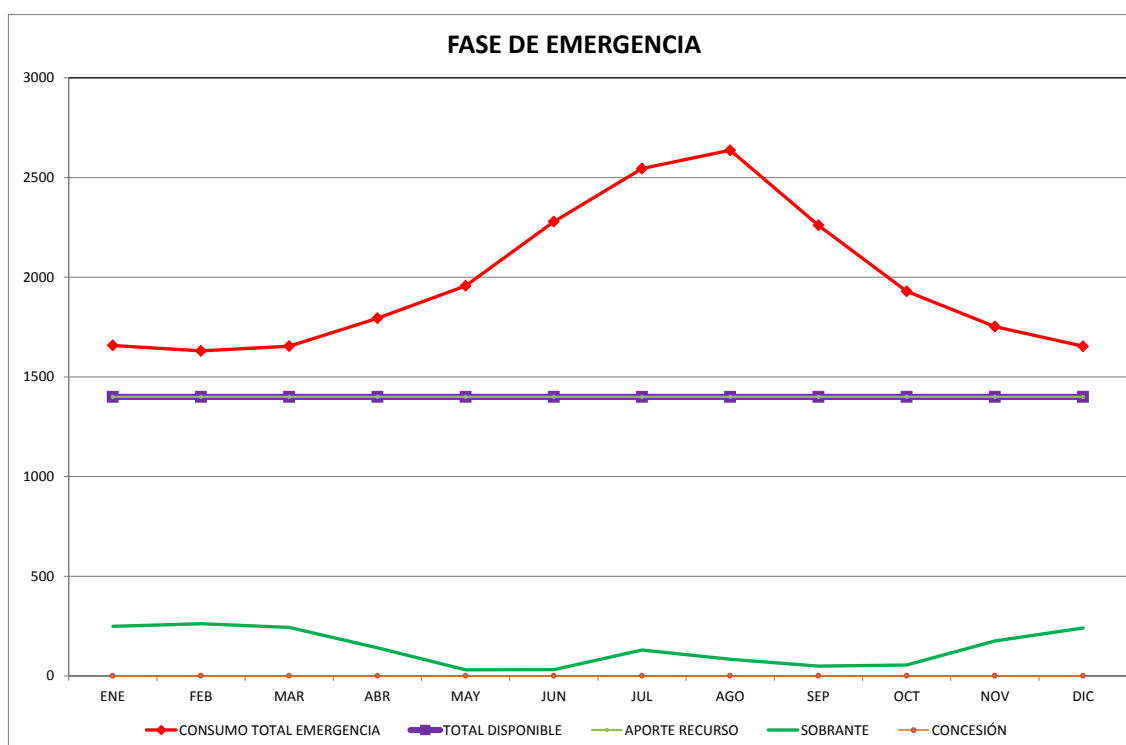
Figura 20. Consumo CAT en fase de emergencia SIN aporte del Ebro y con 100% del recurso disponible
