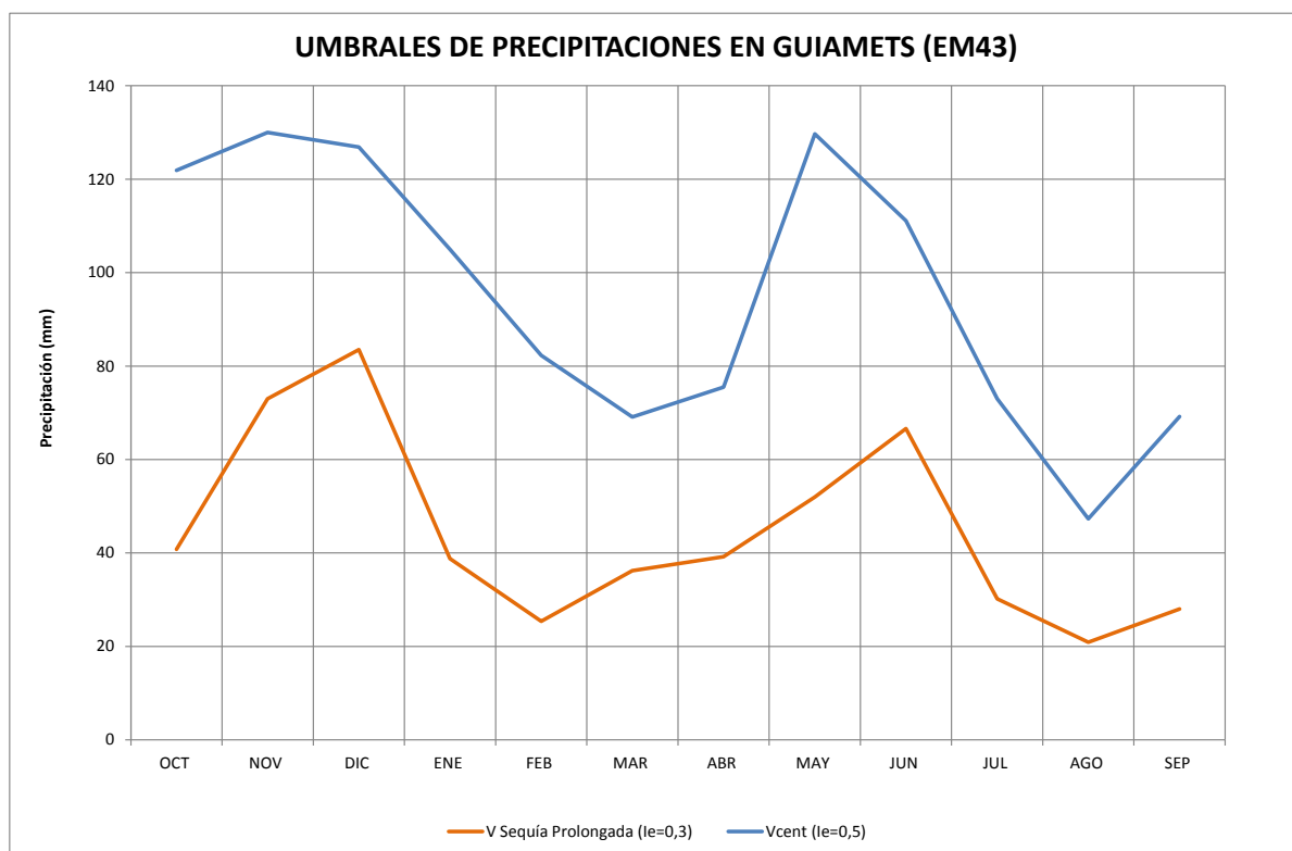
Figura 23. Umbrales de precipitaciones en Guiamets
