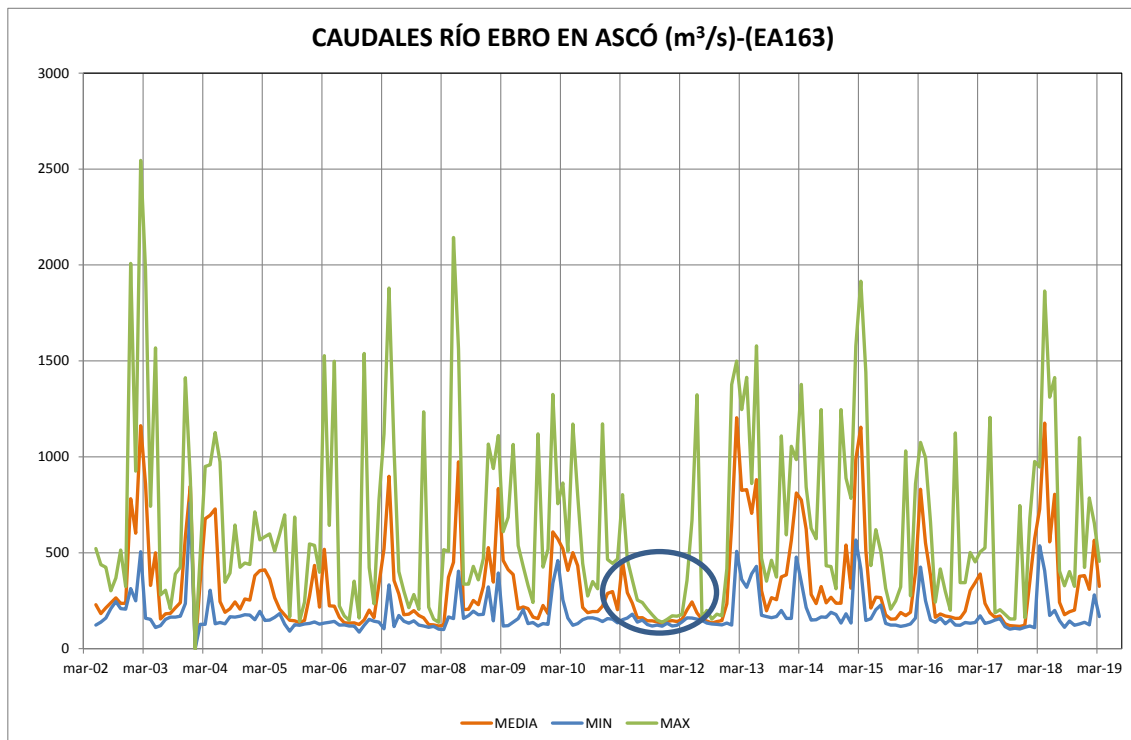
Figura 24. Caudales rio Ebro en Ascó (EA-163)
