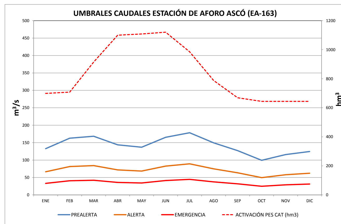
Figura 27. Umbrales Estación de Aforo río Ebro en Ascó (EA-163)
