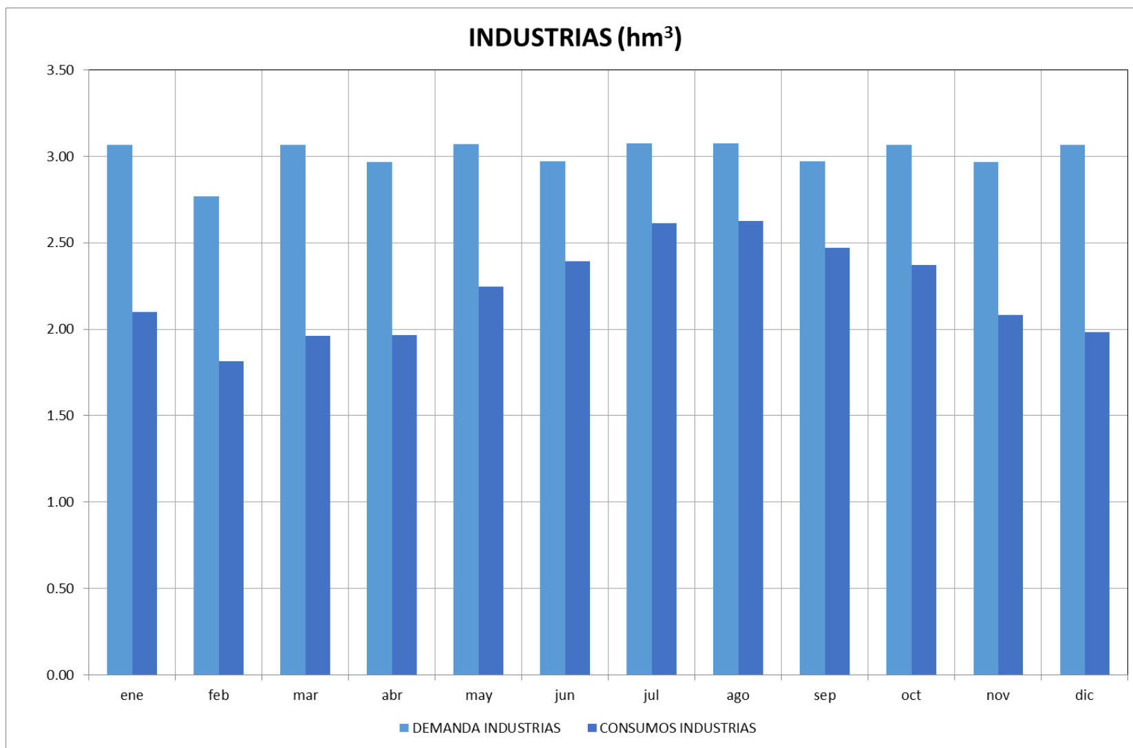
Figura 16. Gráfico de evolución consumos industrias
