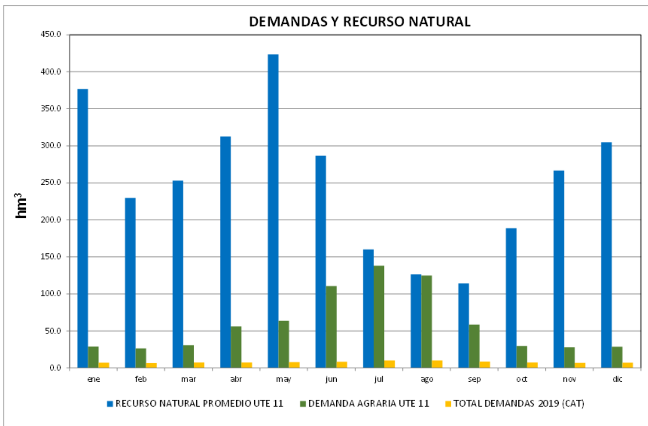
Figura 17. Demanda y recurso natural
