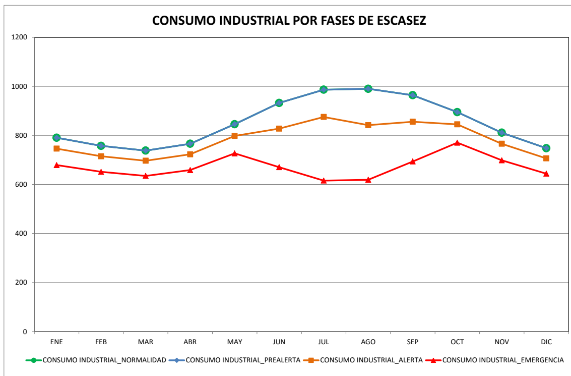
Figura 19. Consumo uso industrial por fases de escasez (l/s)
