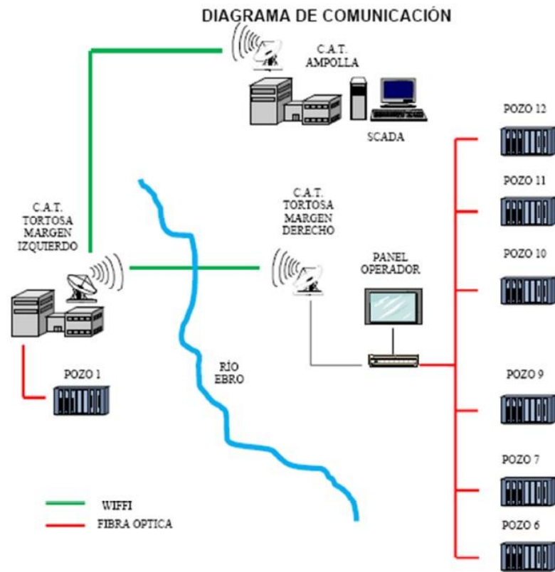
Figura 9. Esquema de comunicació de los pozos de emergencia
