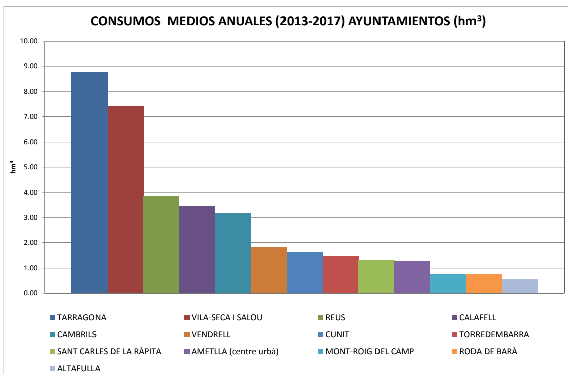
Figura 6. Consumos de ayuntamientos > 0,5 hm 3
