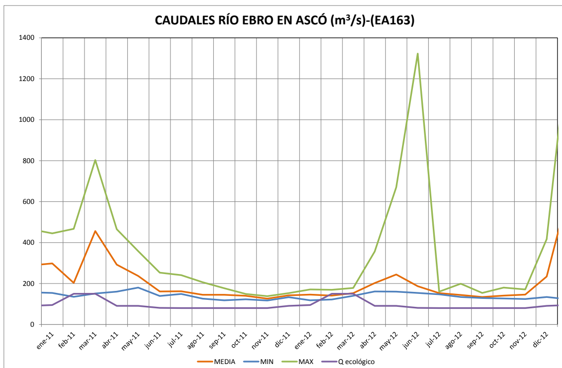
Figura 25. Caudales rio Ebro en Ascó (EA-163), detalle del periodo 2011-2012
