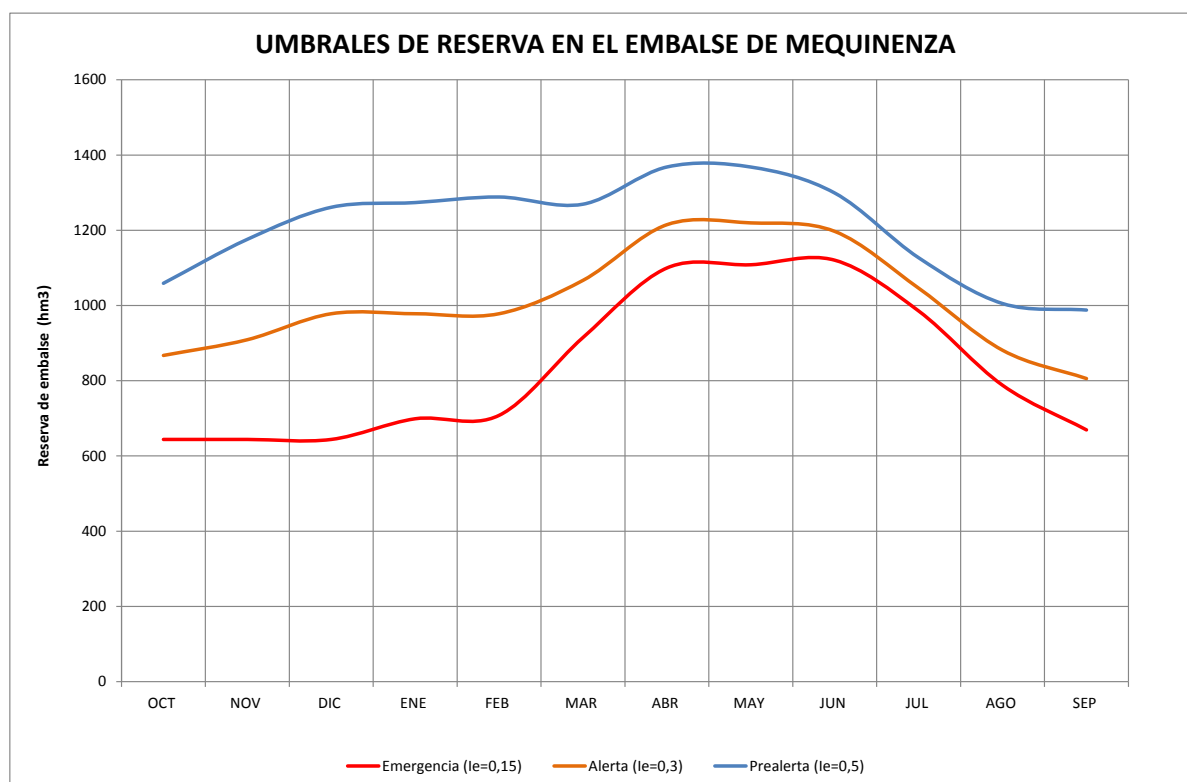
Figura 21. Umbrales de reserva en el embalse de Mequinena
